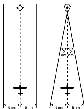
CDI Comparison: GPS vs. VOR
